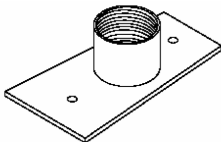
Рис.2. Кабельный адаптер
